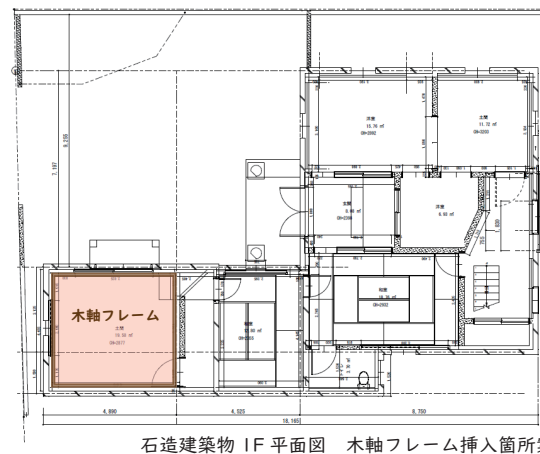
石造建築物 1F 平面図 木軸フレーム挿入箇所案
